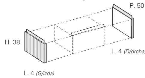
Côtés terminaux Sp.4 cm Costados terminales Sp.4 cm
