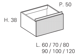
Bases lavabos suspendues H. 38 Bases lavabos suspendidas H. 38
