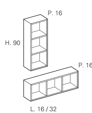
Meubles hauts Ouvertes Módulos altos Abiertos
